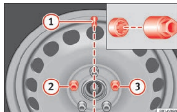
Fig. 82 Changement de roue : valve du pneu (1) et emplacement de montage du boulon de roue antivol (2) ou (3).
