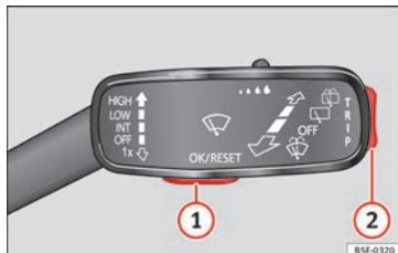
Fig. 45 Levier d'essuie-glace : touches de contrôle.
