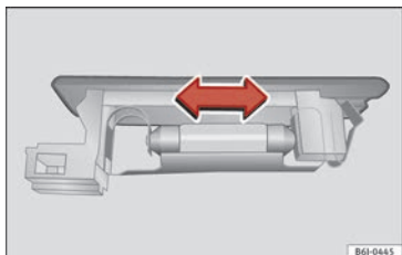
Fig. 119 Éclairage du coffre à bagages.
