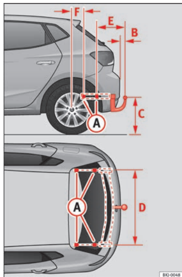
Fig. 221 Points de fixation du dispositif de remorquage.
