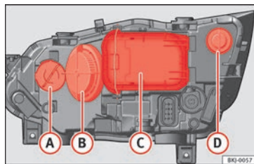
Fig. 109 Projecteur principal halogène
