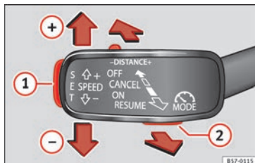
Fig. 183 À gauche de la colonne de direction : troisième levier pour utiliser le limiteur de vitesse.
