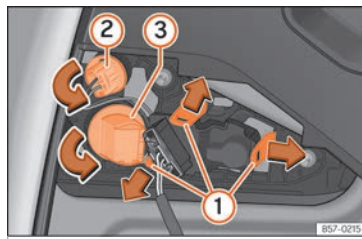
Fig. 117 Démontez le porte-ampoule.
