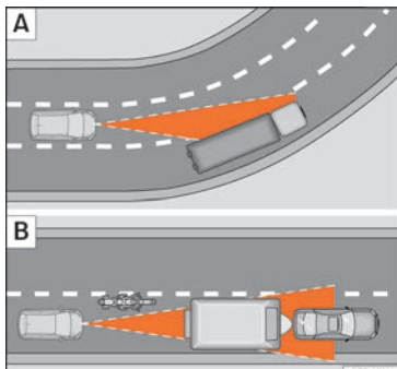
Fig. 264 (A) Véhicule à l'abord d'un virage. (B) Motocycliste circulant à l'avant hors du rayon d'action du capteur radar.
