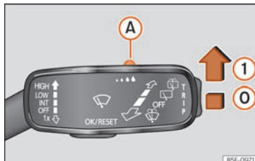
Fig. 156 Levier d'essuie-glace : régler le détecteur de pluie A .
