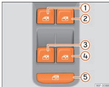
Fig. 147 Détail de la porte du conducteur : commandes des fenêtres.
