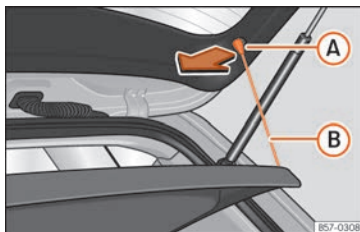
Fig. 170 Dans le coffre à bagages : dépose et repose de la plage arrière.
