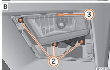
Fig. 112 Phare antibrouillard : enlever la grille.
