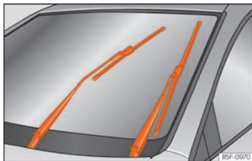
Fig. 84 Essuie-glace en position d'entretien.
