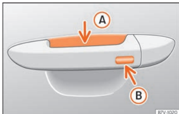
Fig. 140 Système de fermeture et de démarrage sans clé Keyless Access : surface sensible A de déverrouillage vers l'intérieur de la poignée de porte, et surface sensible B de verrouillage vers l'extérieur de la poignée de porte.
